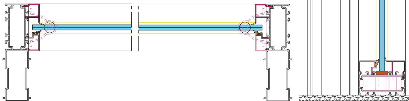
Coupe horizontale
