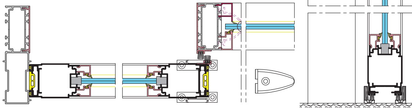
Coupe horizontale
