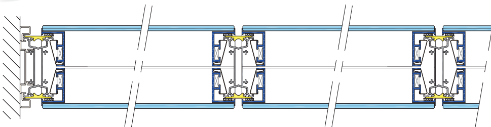
Coupe horizontale
