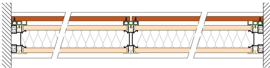
Coupe horizontale
