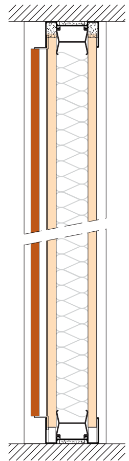
Coupe verticale
