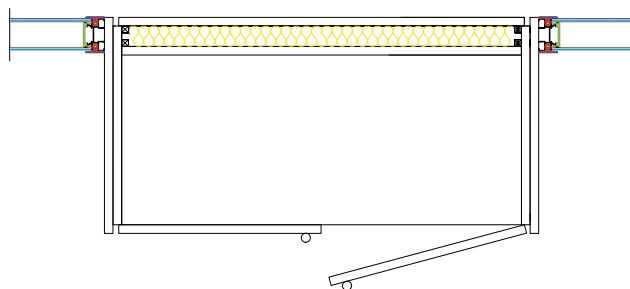
Coupe horizontale
